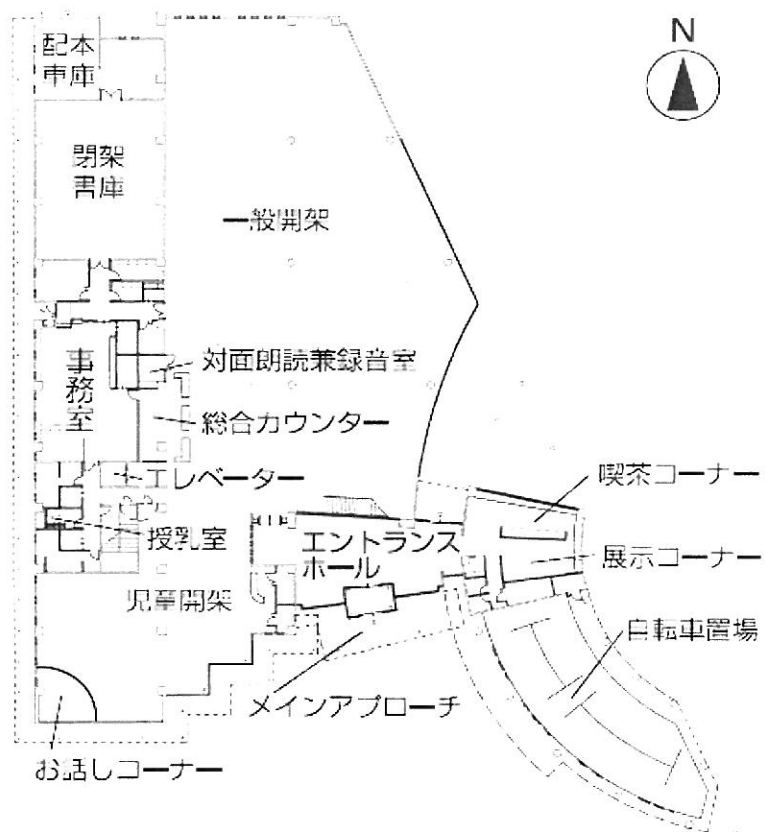
1階平面図
